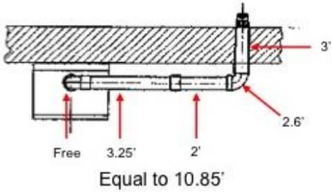
PAHVK Vent Kit
